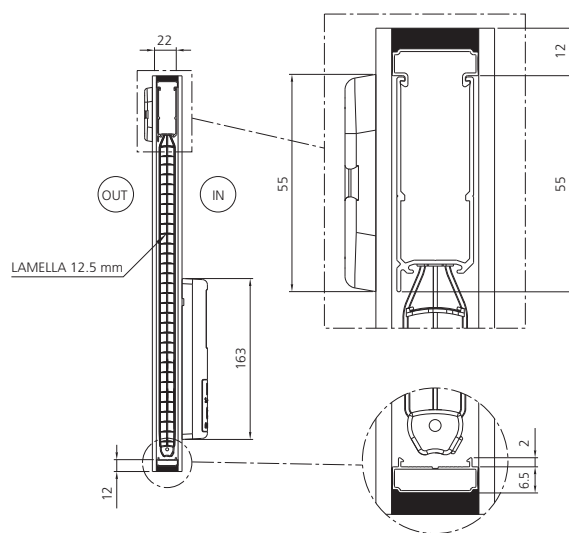
CANALINA ESTRUSA RIBASSATA CON INCASTRO
