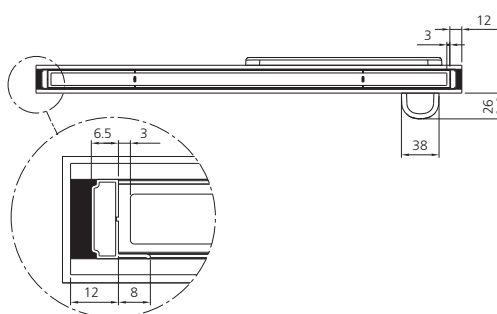
CANALINA ESTRUSA RIBASSATA CON ALETTA
