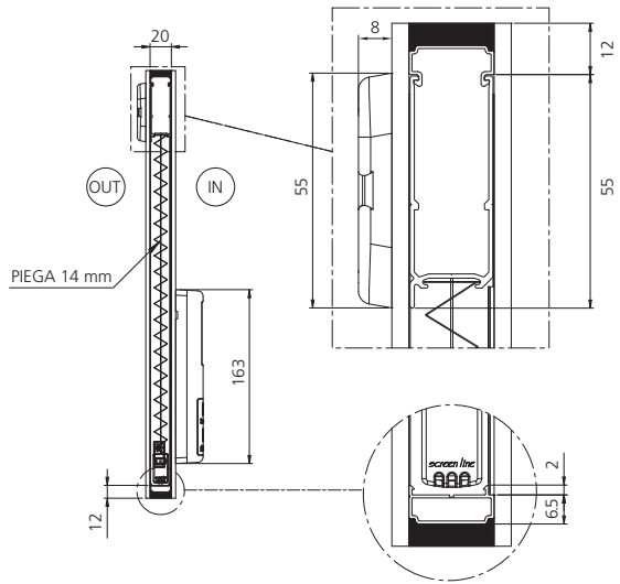
CANALINA ESTRUSA RIBASSATA CON INCASTRO
