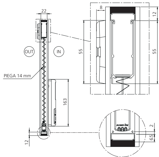
CANALINA ESTRUSA RIBASSATA CON INCASTRO
