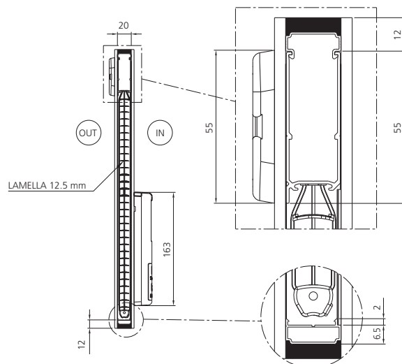
CANALINA ESTRUSA RIBASSATA CON INCASTRO
